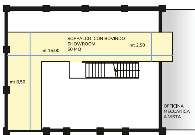
SOPPALCO
